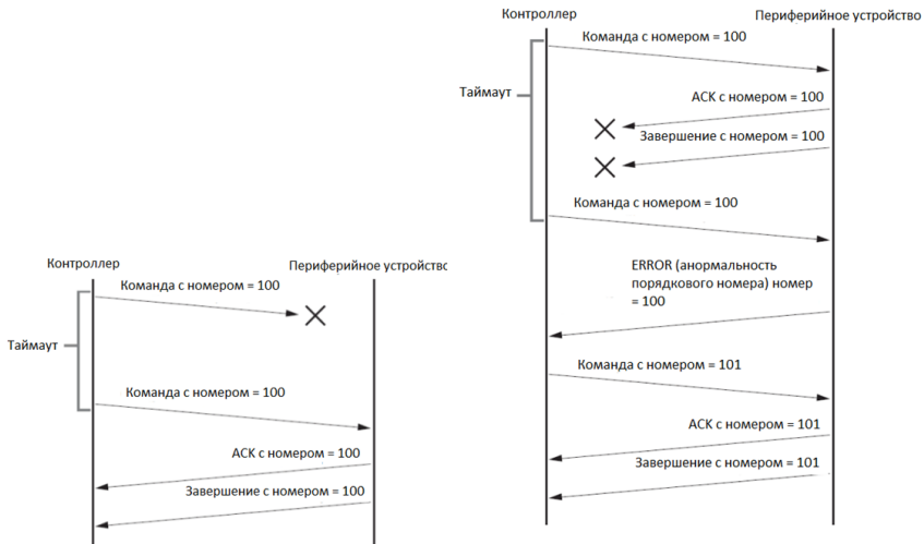
Схема последовательности операций при потере команды
